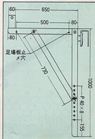
寸法図
