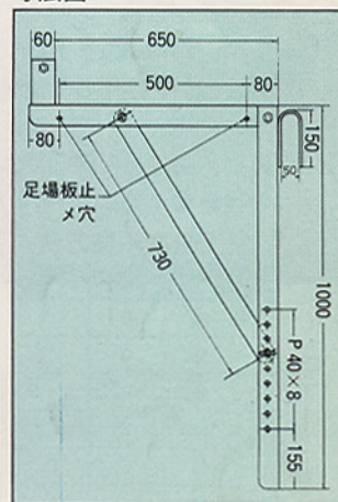
寸法図
